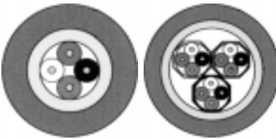
4- ja 12-kuituisen kaapelin rakenne
